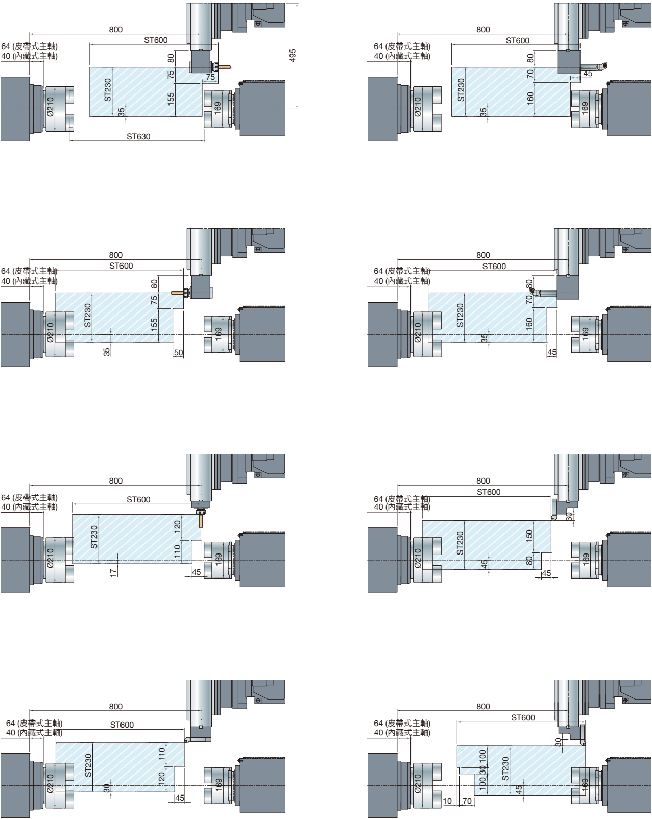
TD-2000YB(C) 16分度/BMT-55刀具
