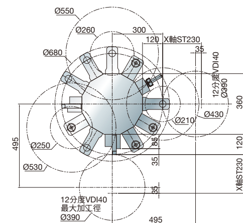
12分度VDI-40刀具
