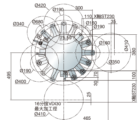
16分度VDI-30刀具
