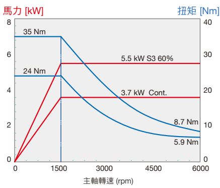
動力刀主軸馬達
