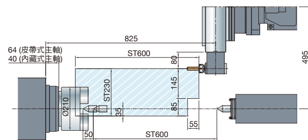
TD-2000Y 16分度/BMT-55刀具
