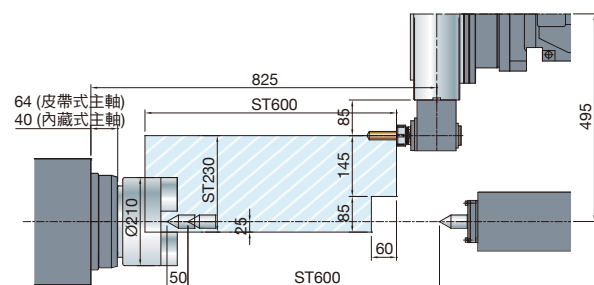
TD-2000Y 12分度/BMT-65刀具
