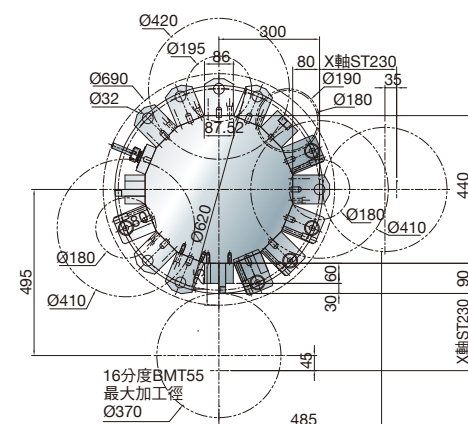
16分度BMT-55刀具
