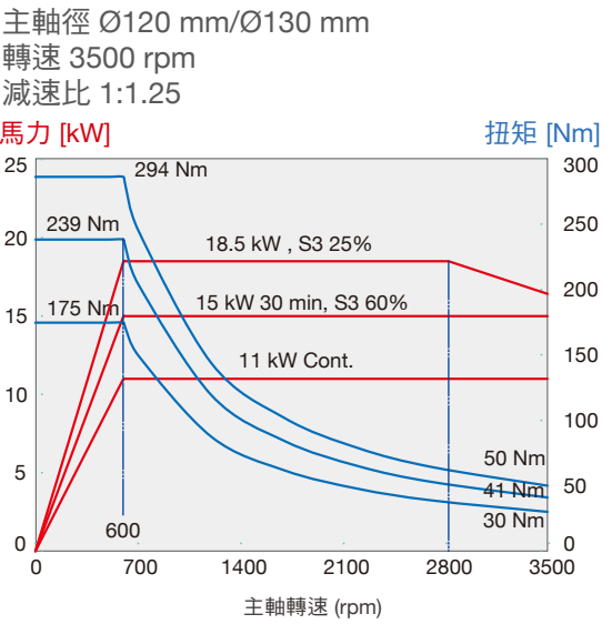
內藏式副主軸馬達 (選配)
