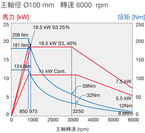
TD-2000Y內藏式主軸馬達 (選配)
