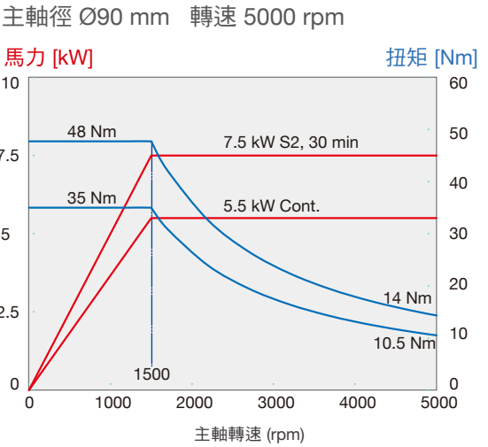
內藏式副主軸馬達 (選配)
