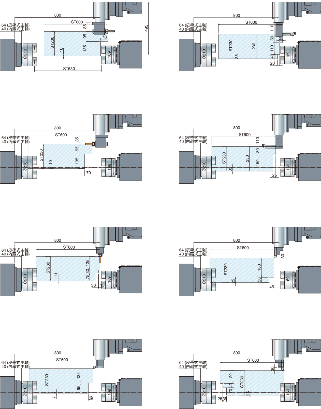
TD-2000YB(C) 16分度/VDI-30刀具
