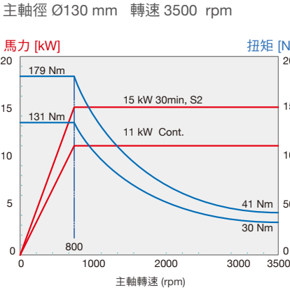
TD-2500Y內藏式主軸馬達 (選配)
