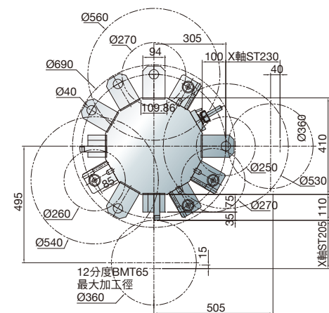
12分度BMT-65刀具
