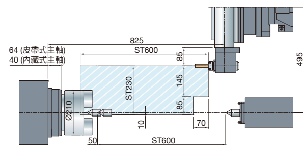
TD-2000Y 16分度/VDI-30刀具
