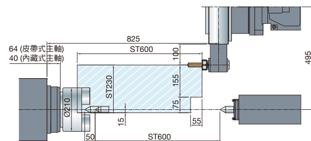
TD-2000Y 12分度/VDI-40刀具
