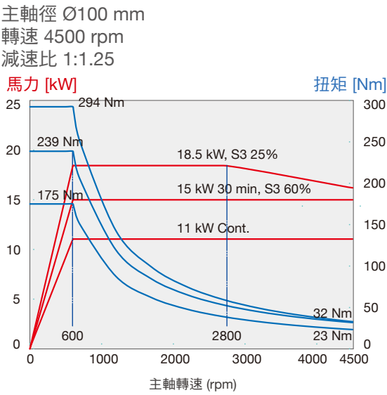
TD-2000Y內藏式主軸馬達 (選配)
