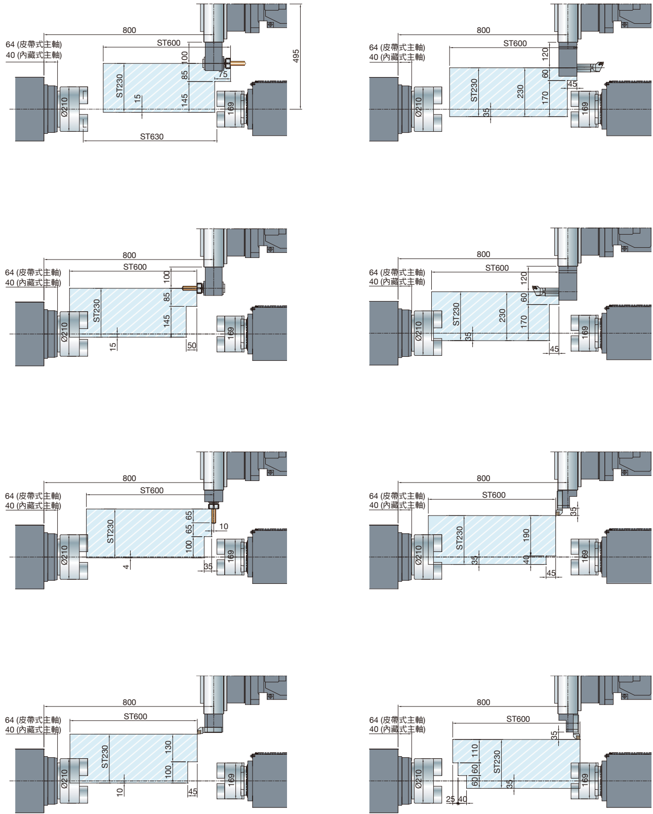
TD-2000YB(C) 12分度/VDI-40刀具
